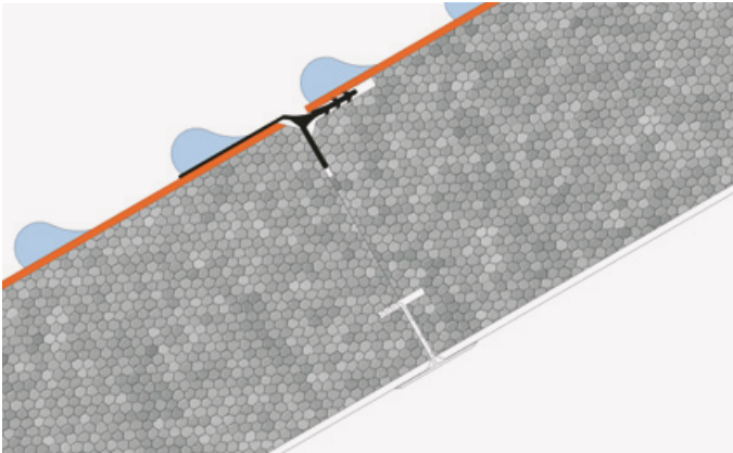
Gegarandeerde afwatering***
