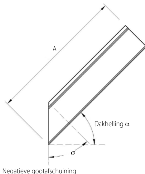
Standaard: recht
