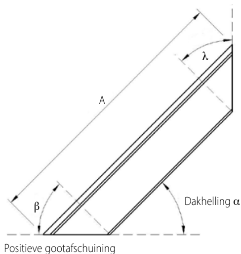
Positieve nokafschuining
