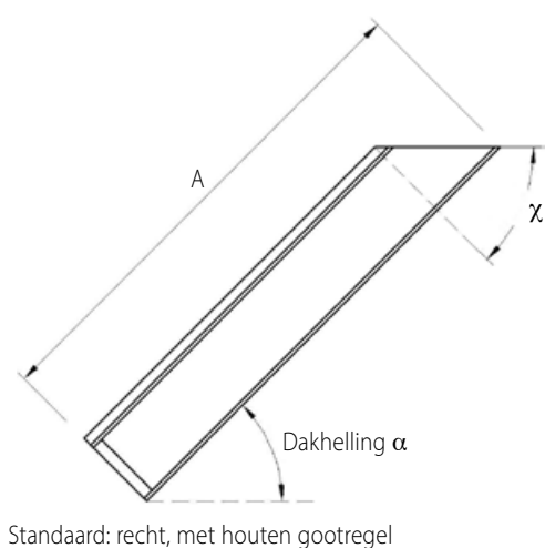
Negatieve nokafschuining
