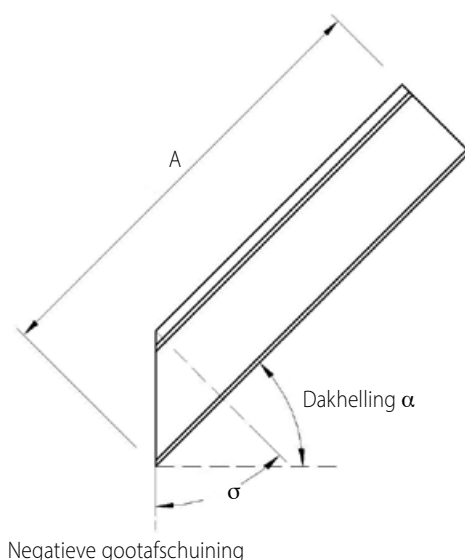
Standaard: recht
